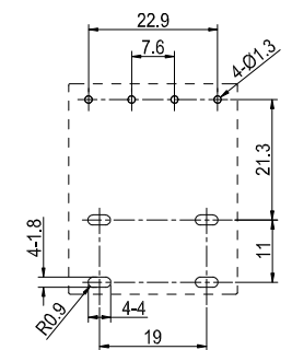
安装尺寸图 (底视图)
