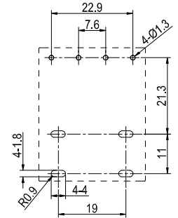
安装尺寸图 (底视图)
